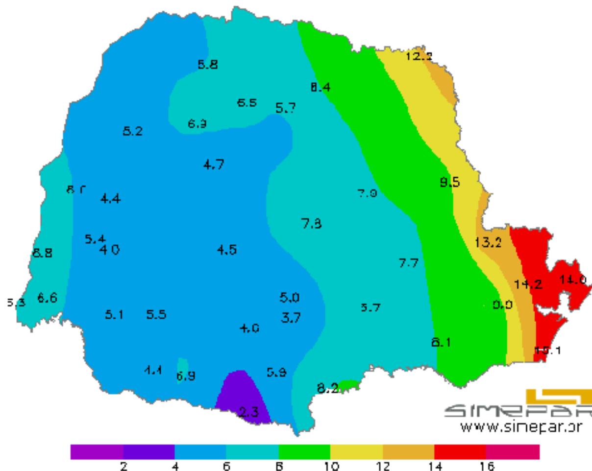
Temperaturas mínimas (°C) Registros até às 08 h de 02/08/2011
