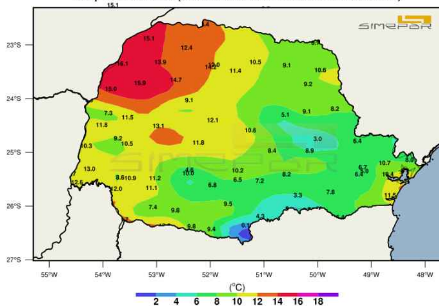
Temperatura Mínima (13/08/2018 00:00h - 13/08/2018 04:15h GMT-3)
